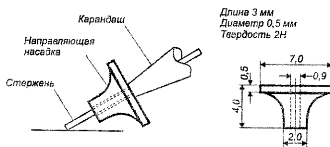
Рисунок 1. Источник Су-Нильсена
