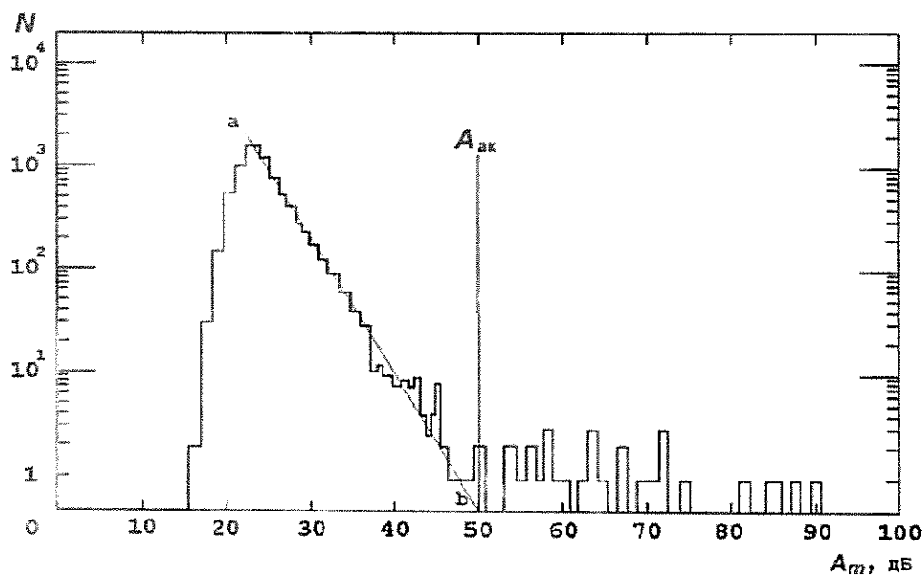
Рисунок П4.2.1. Дифференциальное распределение амплитуд импульсов акустической эмиссии для стали марки 15Х2НМФА
