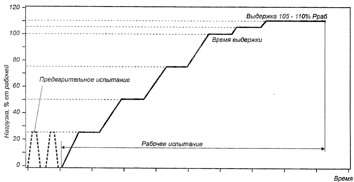
Рисунок ПЗ.2. Рекомендуемый график нагружения при АЭ сопровождении гидравлического испытания резервуаров
