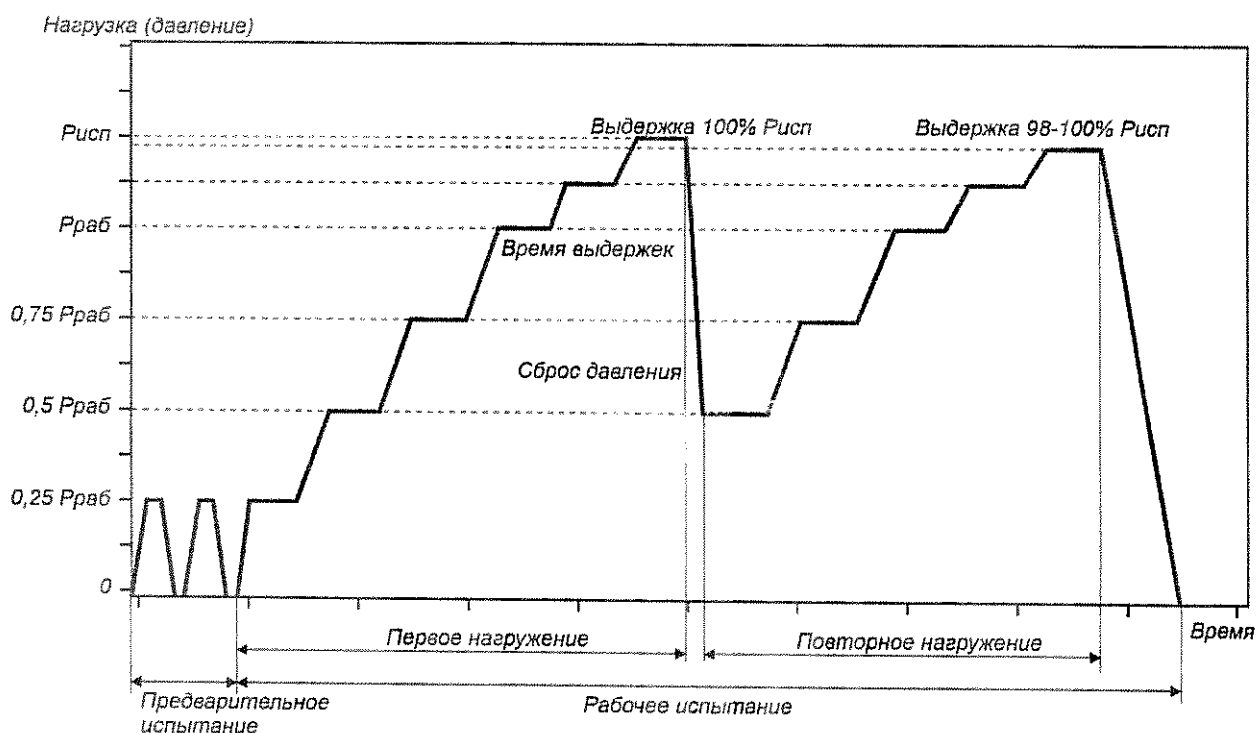
Рисунок ПЗ.1. Рекомендуемый график нагружения объектов контроля
