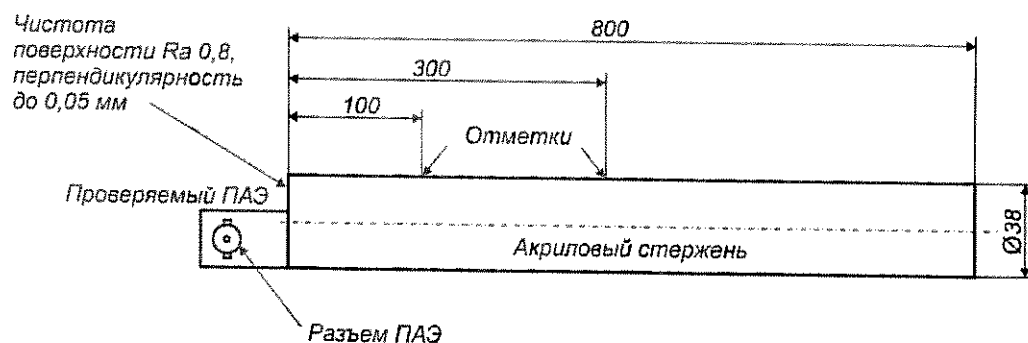
Рисунок 2. Проверка ПАЭ с помощью акрилового стержня
